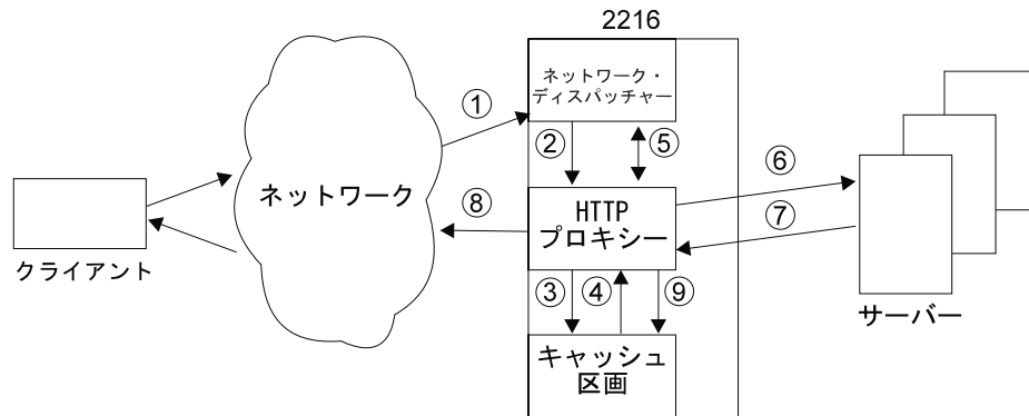
図10. Web サーバー・キャッシュが存在し、キャッシュでヒットしない場合のネットワーク・ディスパッチャー
