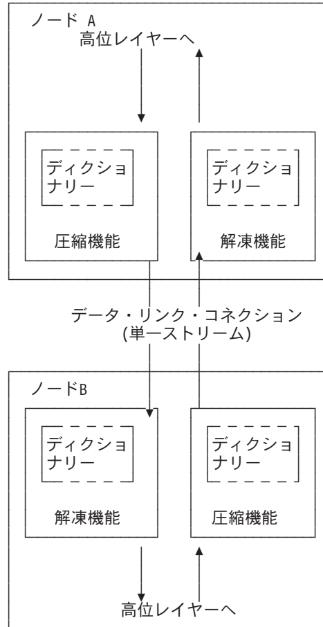
図 12. データ・ディクショナリーを使用した双方向データ圧縮の例
