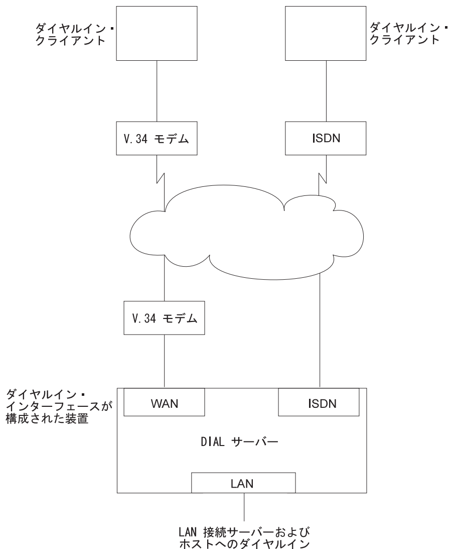
図23. ダイヤルインをサポートする DIAL サーバーの例
