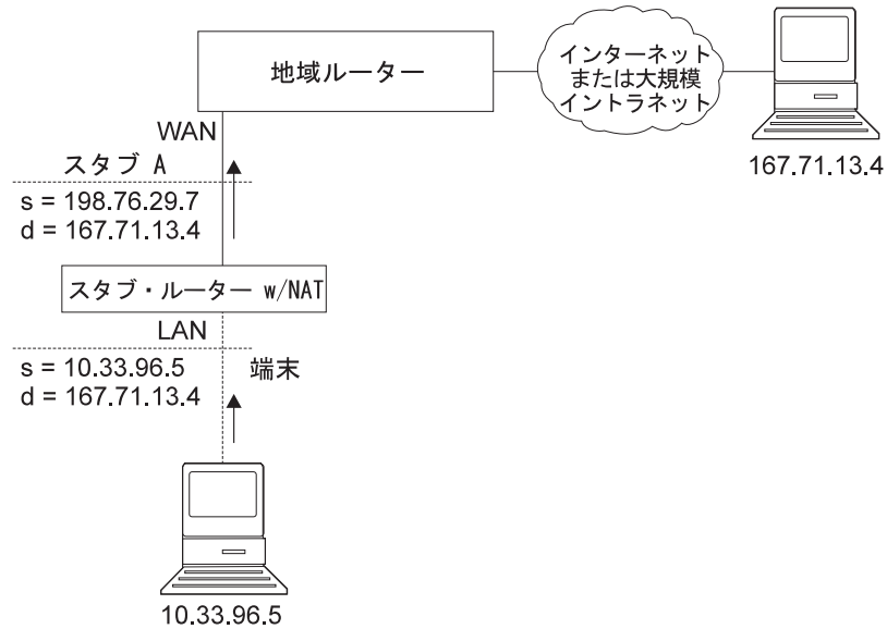
図 21. NAT を実行するネットワーク
