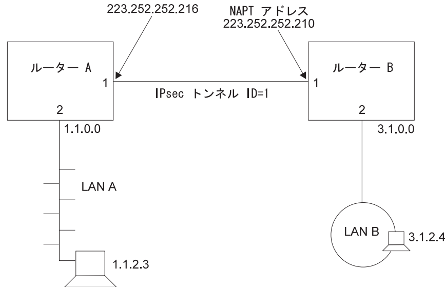
図 19. IPsec と NAT を備えたルーター
