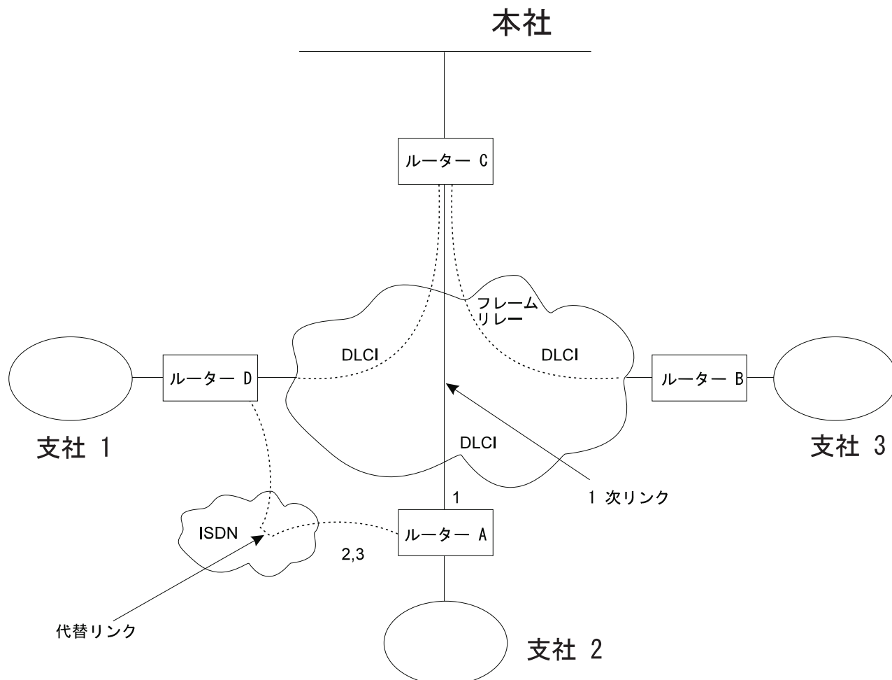
図4. サンプル WAN 再ルート構成. 支社はフレーム・リレーを使用して本社に接続。
