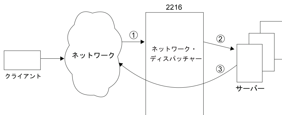
図9. Web サーバー・キャッシュが存在しない場合のネットワーク・ディスパッチャー
