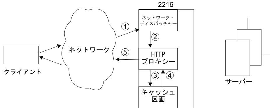
図 11. Web サーバー・キャッシュが存在し、キャッシュでヒットする場合のネットワーク・ディスパッチャー
