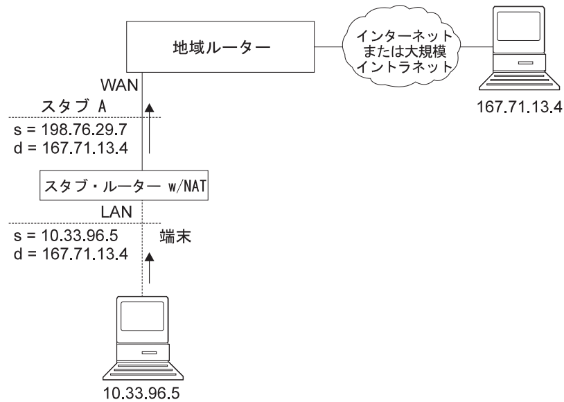
図22. NAT を実行するネットワーク
